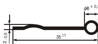
№ 07320902 Тегло: 72 g/m Hardness acc. Shore °A - 75 ±5
